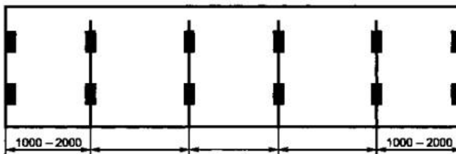
Рисунок В.7 - Контейнеры типов 1ЕЕ, 1АА, 1А или 1АХ (без тоннеля для установки на полуприцепе с передней балкой типа «шея гуся»).
