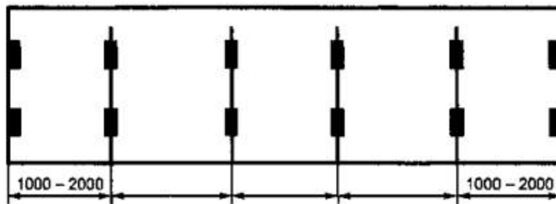
Рисунок В.5 - Контейнеры типов 1ВВВ, 1ВВ, 1В или 1ВХ.
