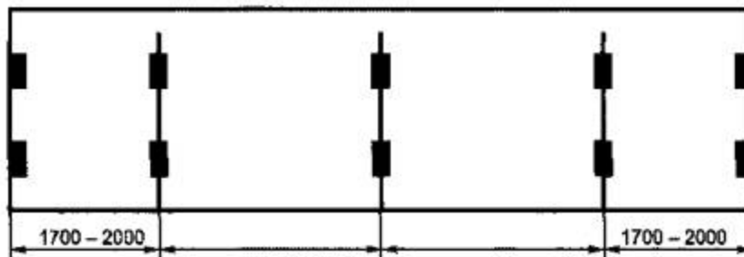
Рисунок В.6 - Контейнеры типов 1ЕЕ, 1АА, 1А или 1АХ (без тоннеля для установки на полуприцепе с передней балкой типа «шея гуся»).
