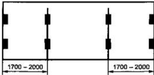
Рисунок В.2 - Контейнеры типов 1СС, 1С или 1СХ.
