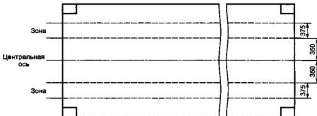
Рисунок В.1 - Основание контейнера
