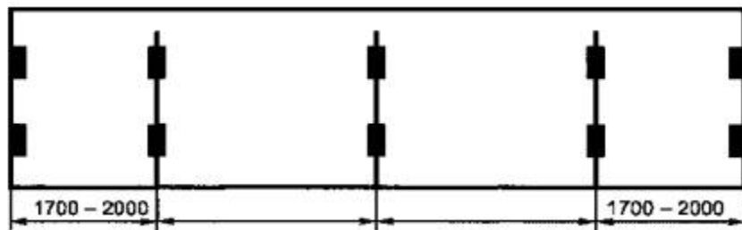
Рисунок В.4 - Контейнеры типов 1ВВВ, 1ВВ, 1В или 1ВХ.
