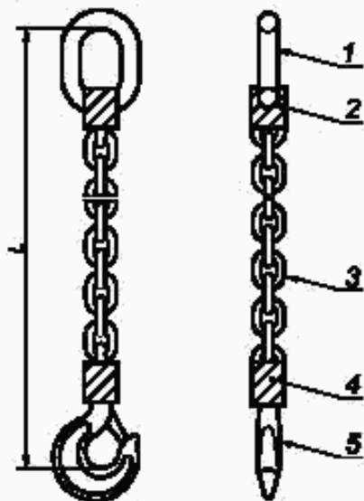
а) Смонтированная стропальная цепь из одного жгута
