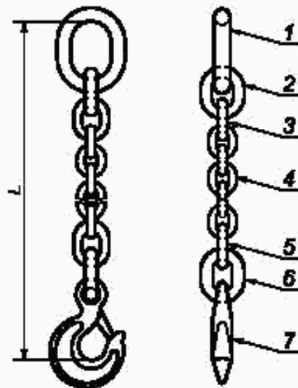
б) Сварная стропальная цепь из одного жгута
